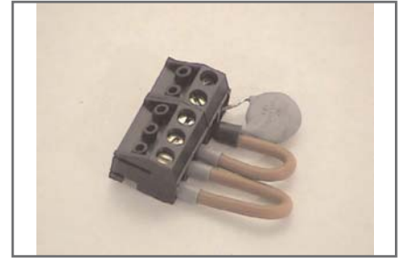
9015.0964 Loom transfo config 115V
